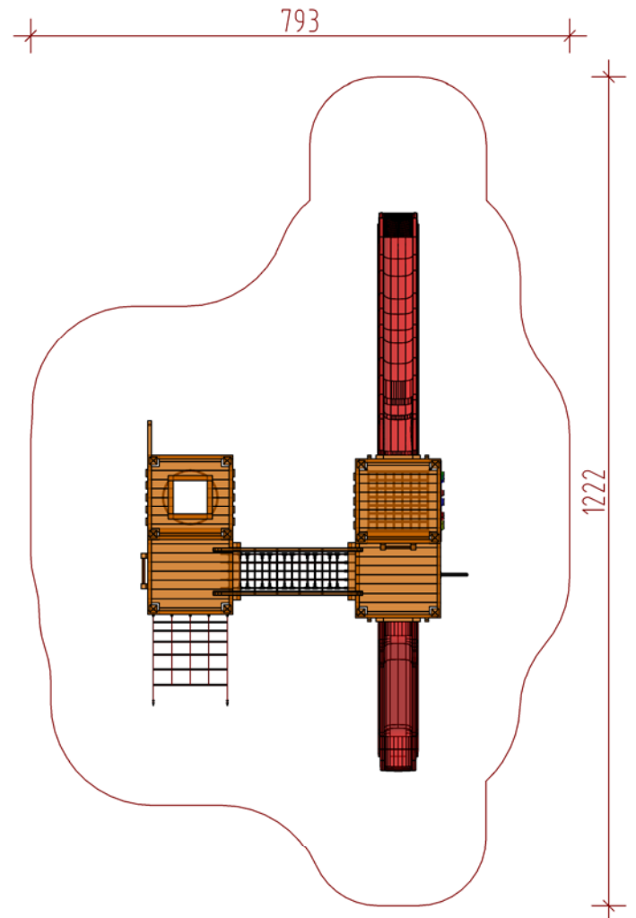
M 1:100 A=67.3m 2
