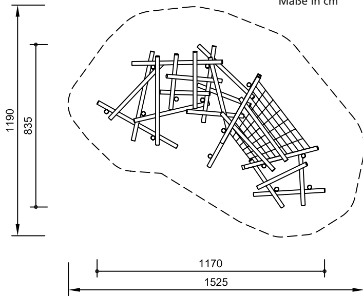
Maßstab 1:200 Maße in cm
